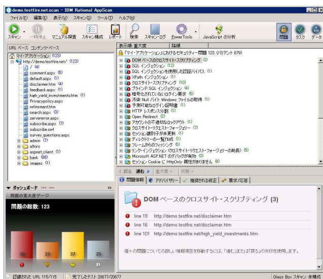
図 1. AppScan のスキャン結果例
